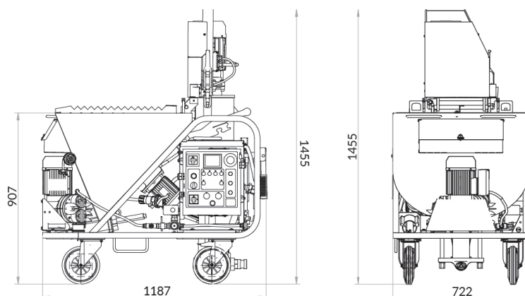
Turbomalaxeur
